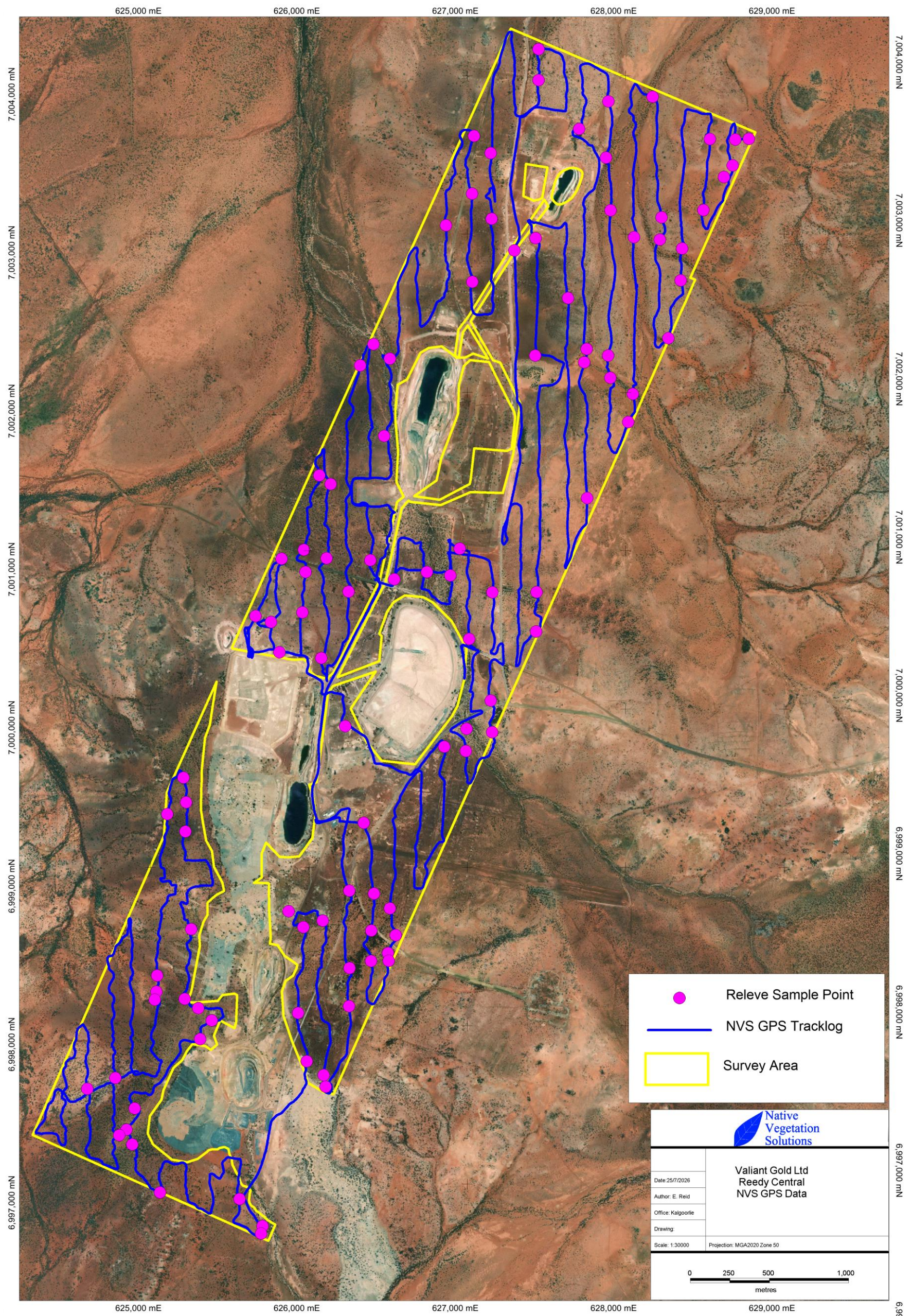
Map 2: NVS GPS Data
